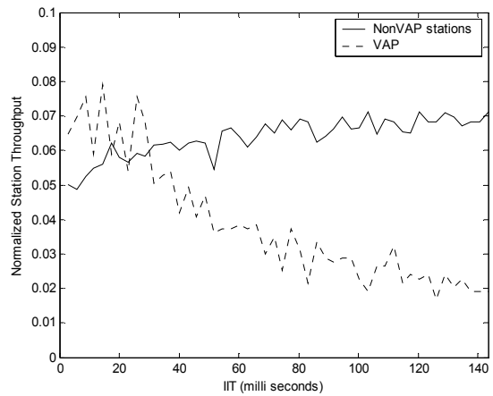
Fig. 7 Optimum IIT value
