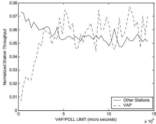
Fig. 8 Optimum VAP/POLL limit value
